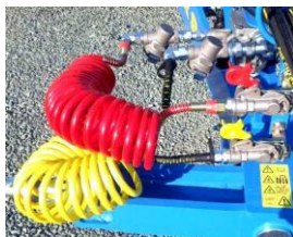
Dviejų žarnų vieno kontūro stabdžiai
